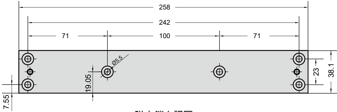
磁力鎖上視圖
