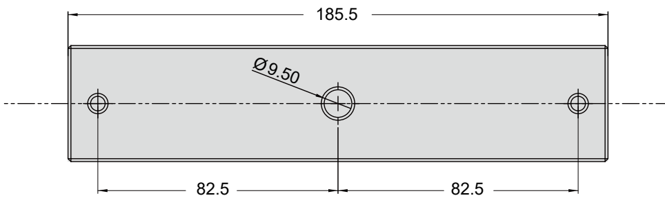
吸附鐵板正視圖
